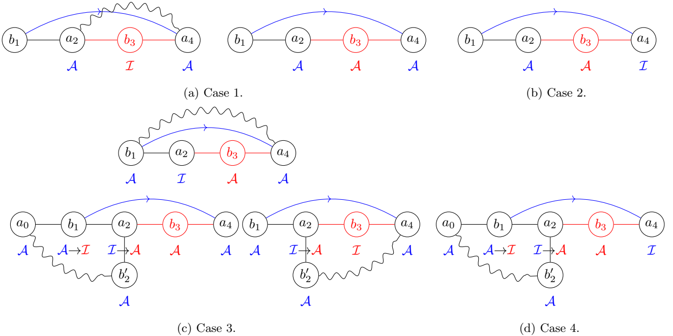
Figure 3: Lemma 18.
