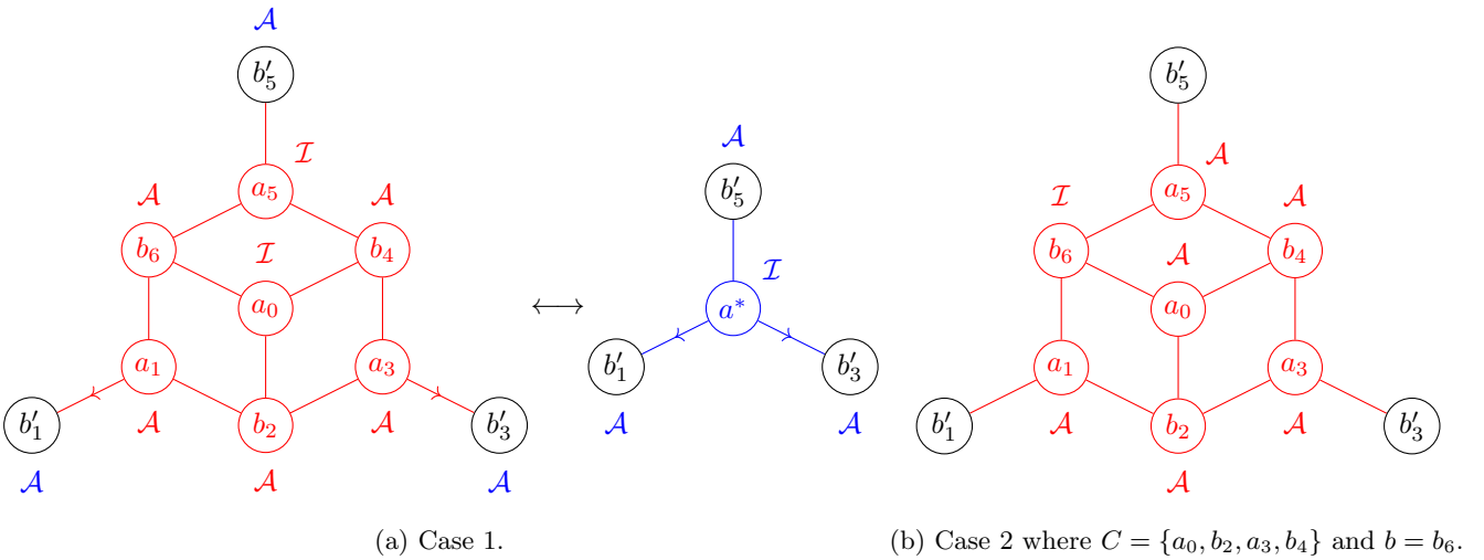
Figure 4: Lemma 19.
