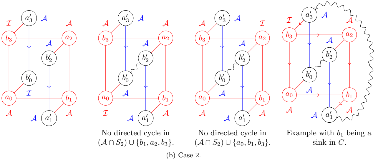
Figure 6: Lemma 21.
